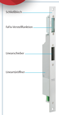
Schließblech
